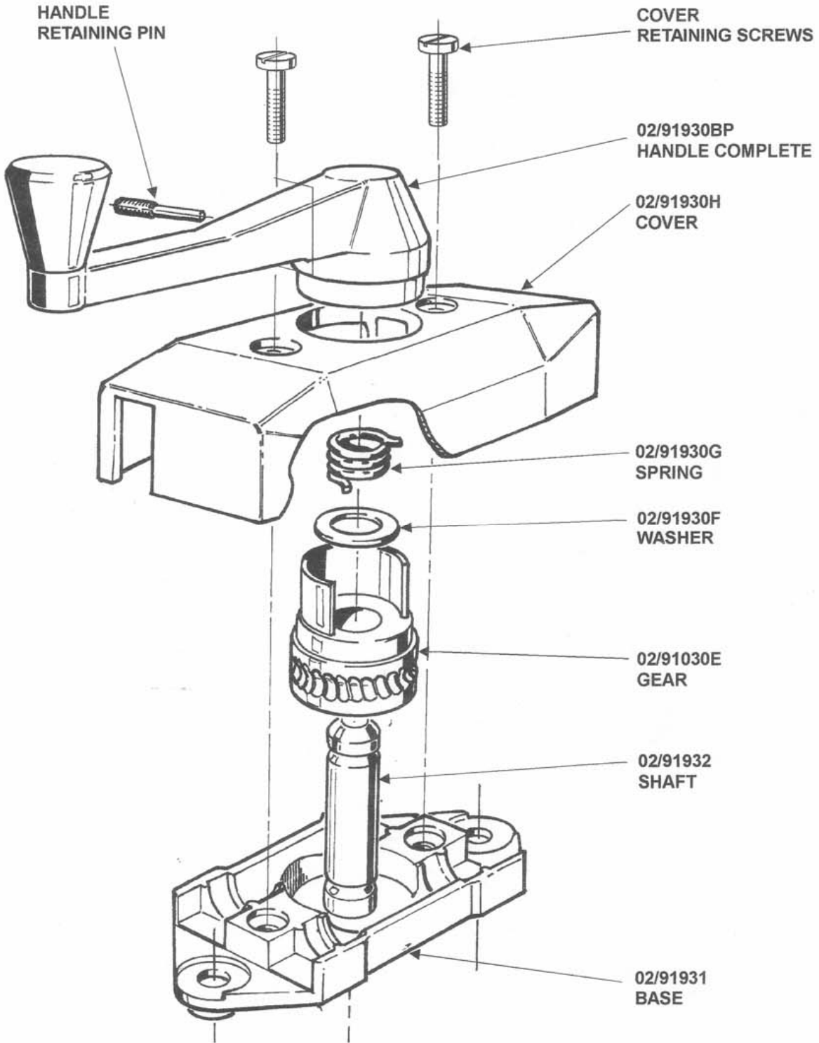
MINI OPERATOR ASSEMBLY 02/101A
